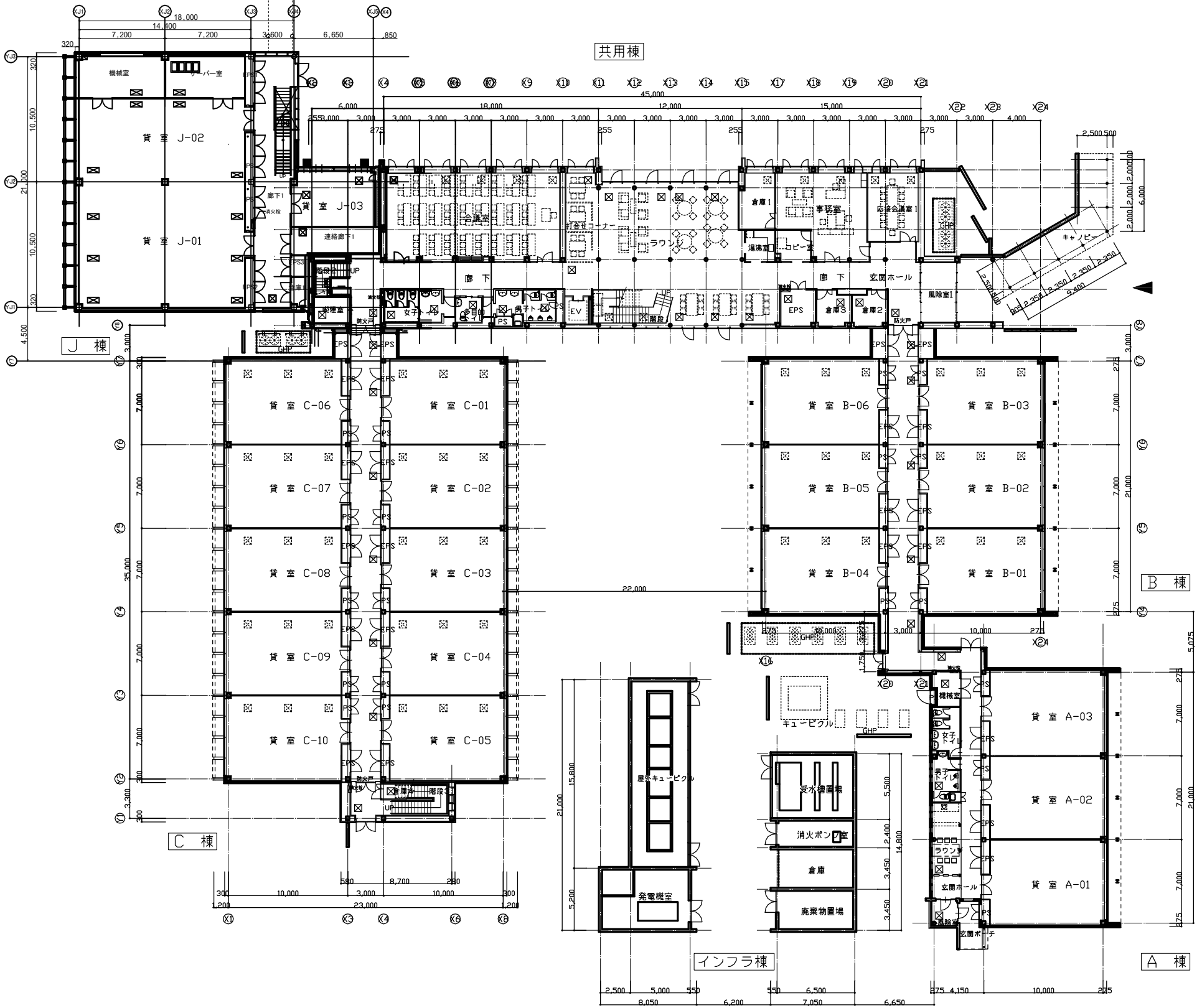
1階平面図
